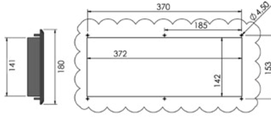
Kesim Ölçüleri / Cutting Dimensions
