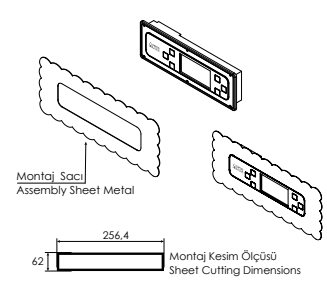
Arka yüzey montaj şekli Backside assembly
