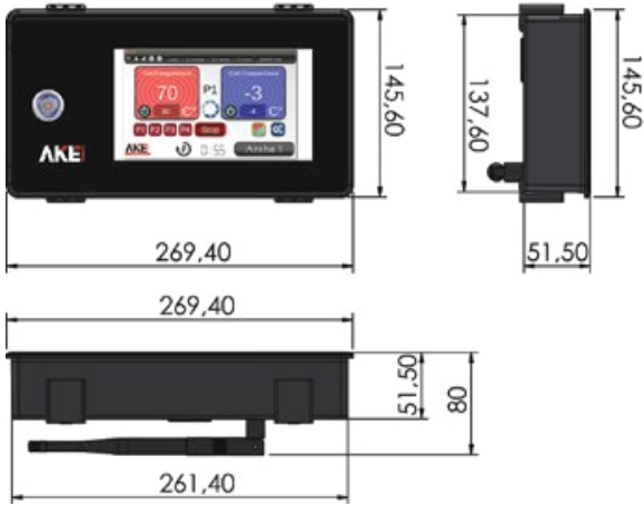
Kesim Ölçüleri / Cutting Dimensions
