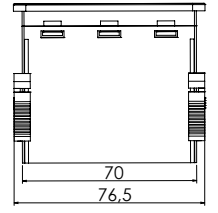
MONTAJ ŞEKLİ/ASSEMBLY TYPE
