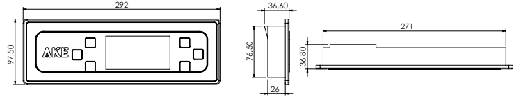
Ön yüzey montaj şekli Front-side assembly
