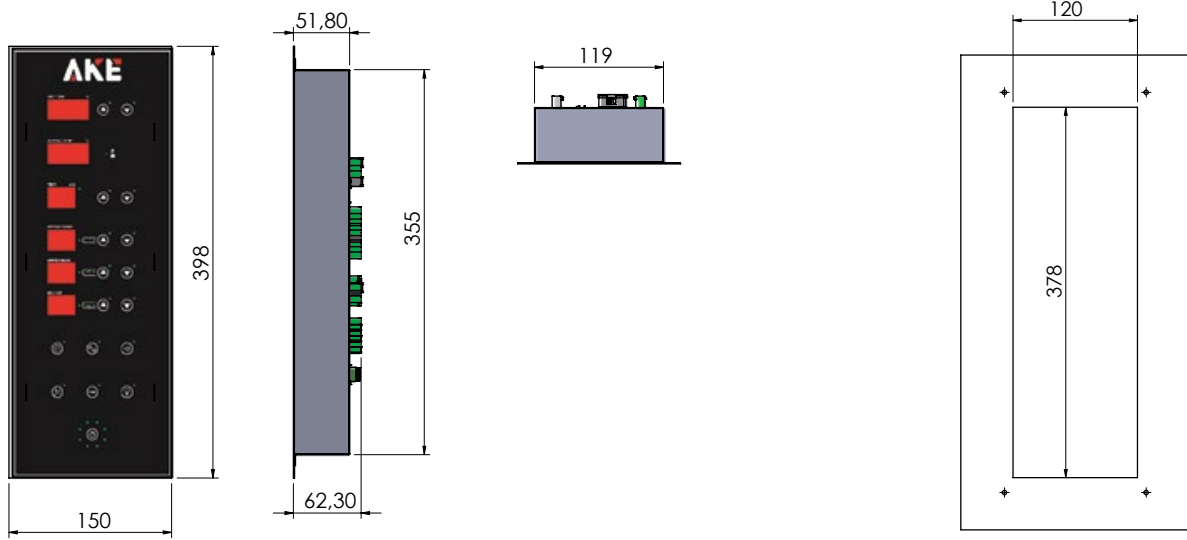
Kesim Ölçüleri / Cutting Dimensions
