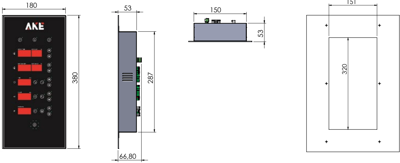
Kesim Ölçüleri / Cutting Dimensions
