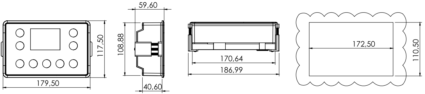
Kesim Ölçüleri / Cutting Dimensions
