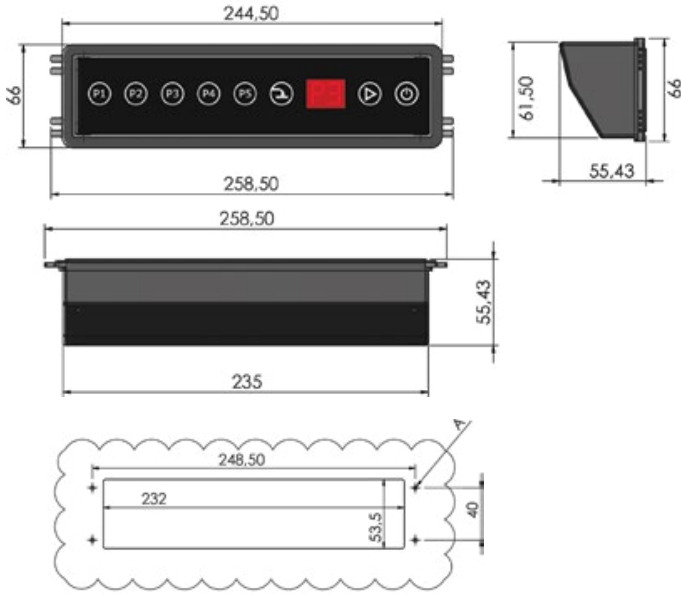
Kesim Ölçüleri / Cutting Dimensions
