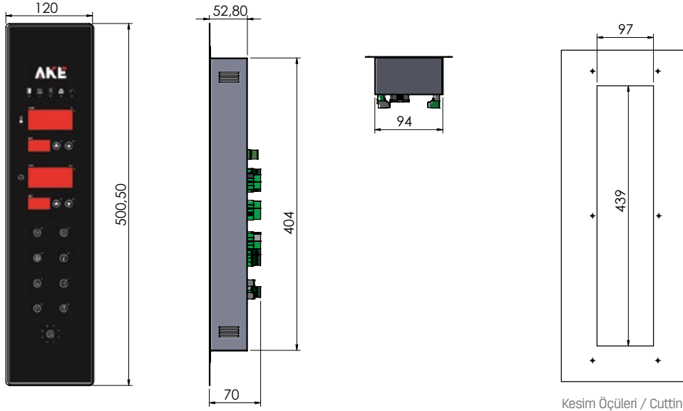
Kesim Ölçüleri / Cutting Dimensions
