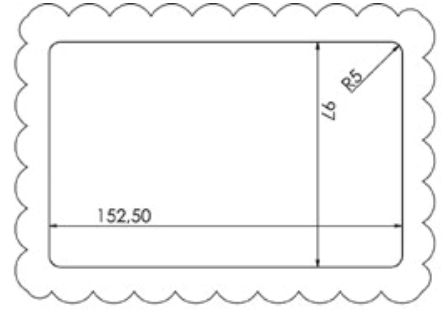
Kesim Ölçüleri / Cutting Dimensions
