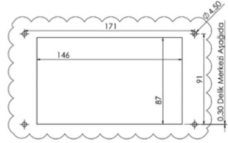
Kesim Ölçüleri / Cutting Dimensions
