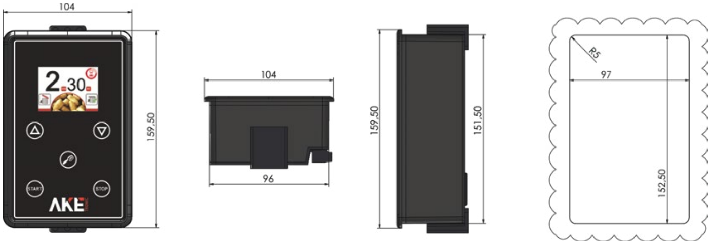
Kesim Ölçüleri / Cutting Dimensions
