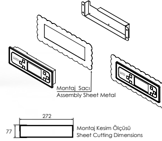
Ön yüzey montaj şekli Front-side assembly
